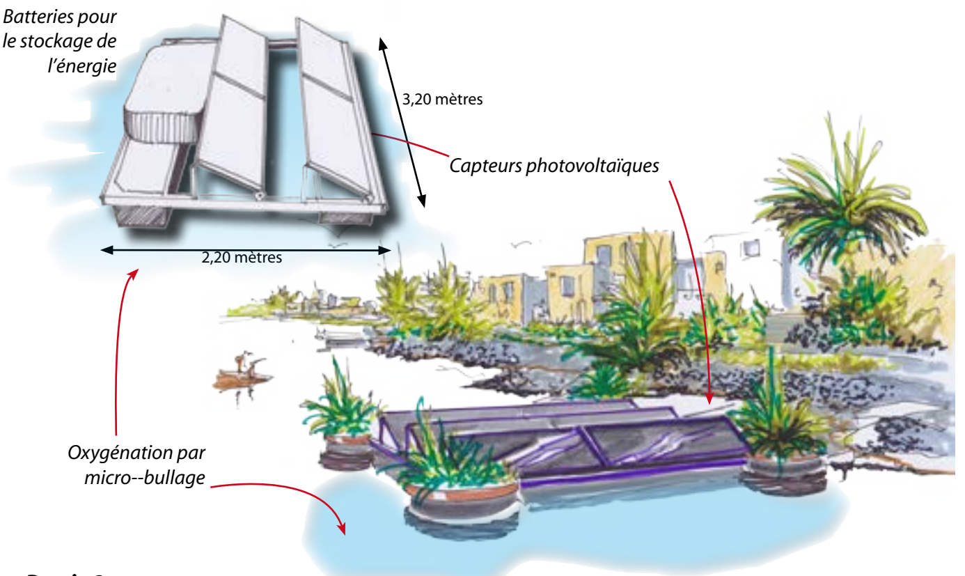
Dessin 2 Structure flottante solaire de traitement de l'eau (type Aquagreen ©)
