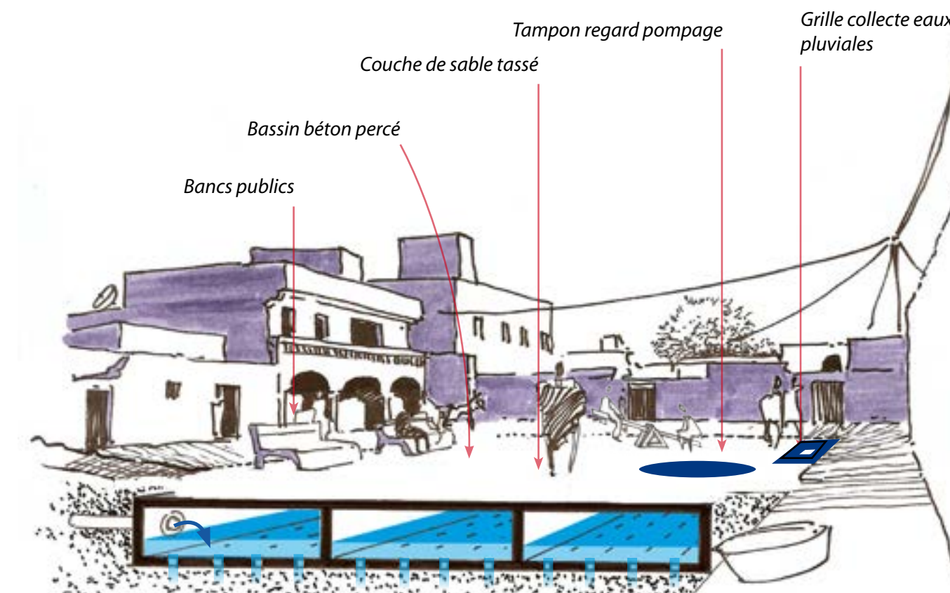
Dessin 2 Stockage des eaux pluviales dans des bassins affleurant en béton percés
