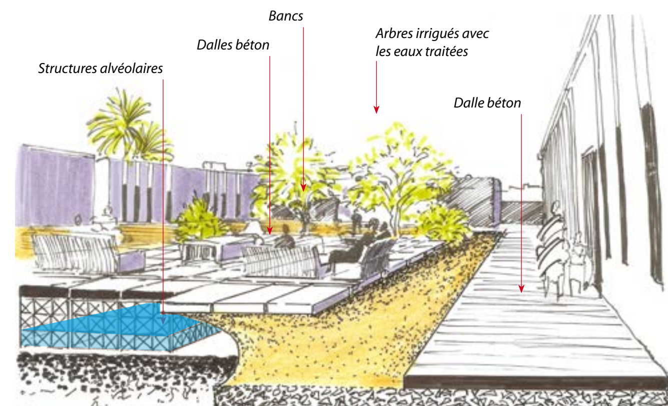
Dessin 2 Bassin de stockage des eaux pluviales équipées de structures alvéolaires
