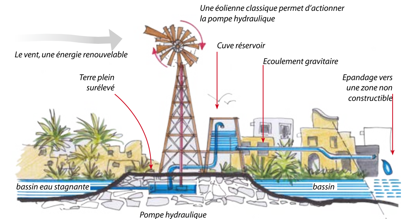
Dessin 1 Evacuation des eaux stagnantes par une pompe hydraulique actionnée par une éolienne
