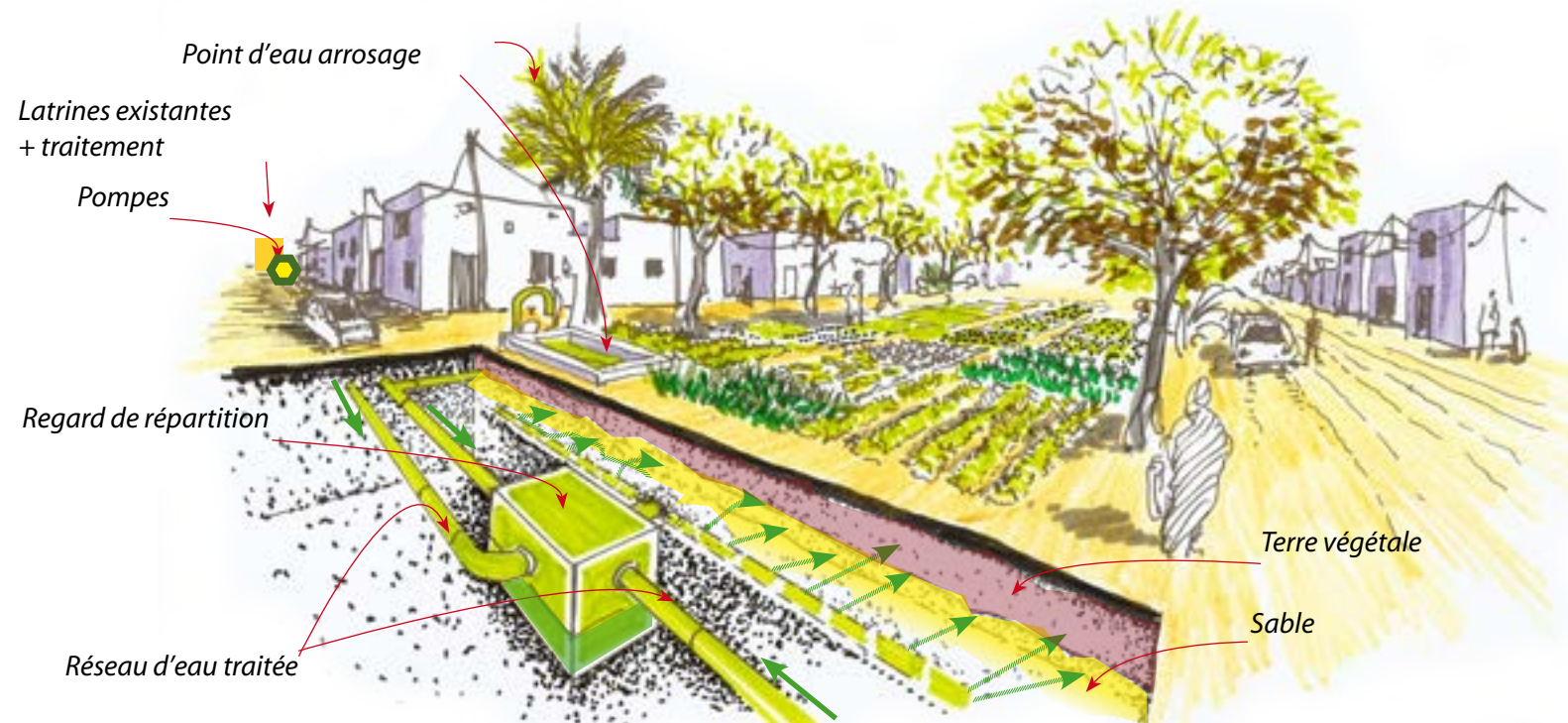
Lit filtrant horizontal pour l'arrosage de jardins maraîchers de quartiers
