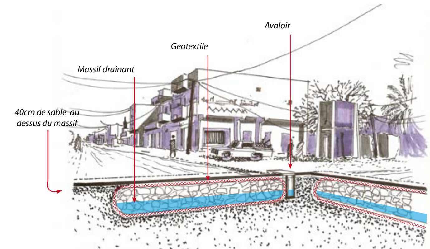
L'eau est stockée par massif drainant Dessin 1
