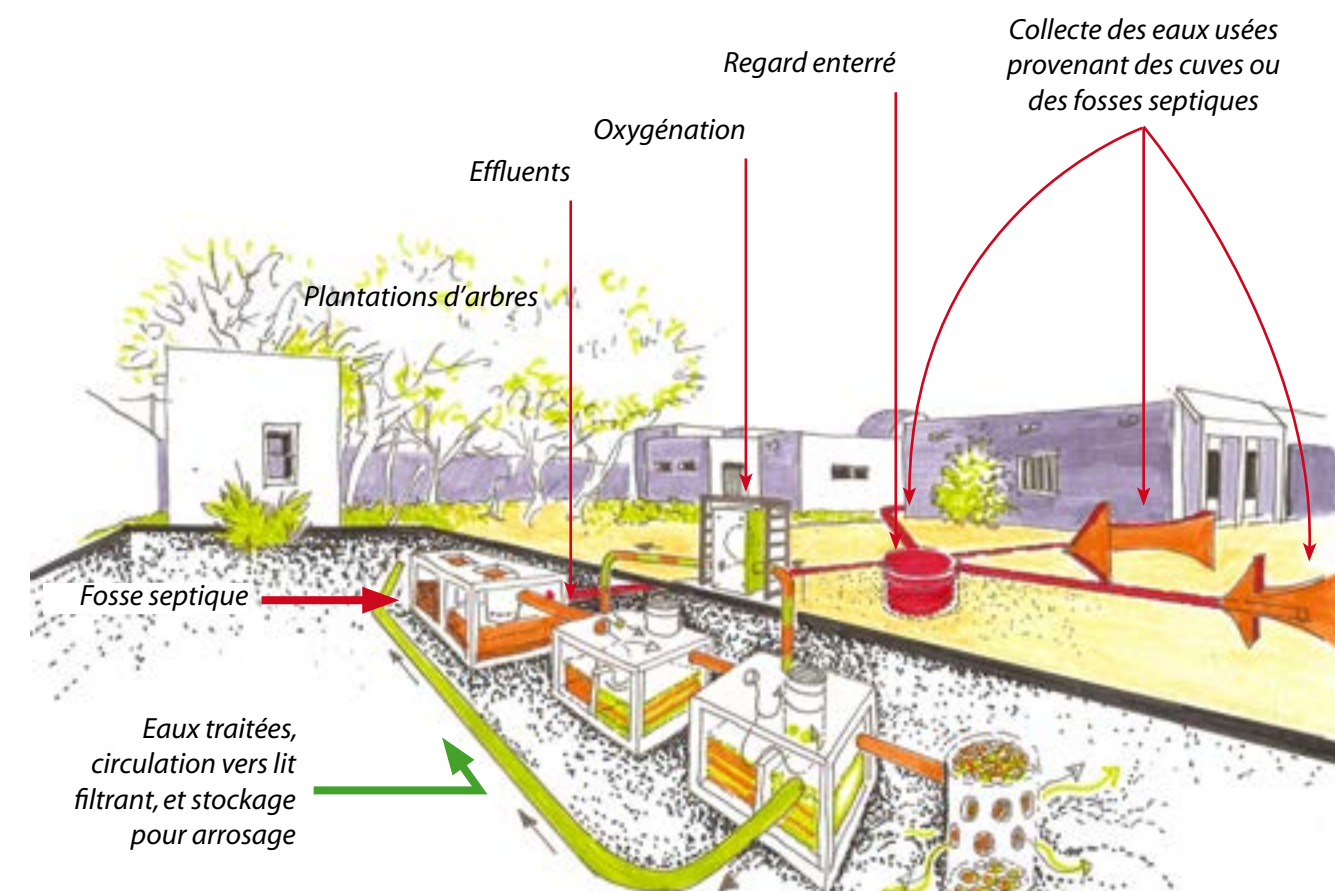
Dessin 2 Traitement des eaux usées pour l'irrigation des plantes
