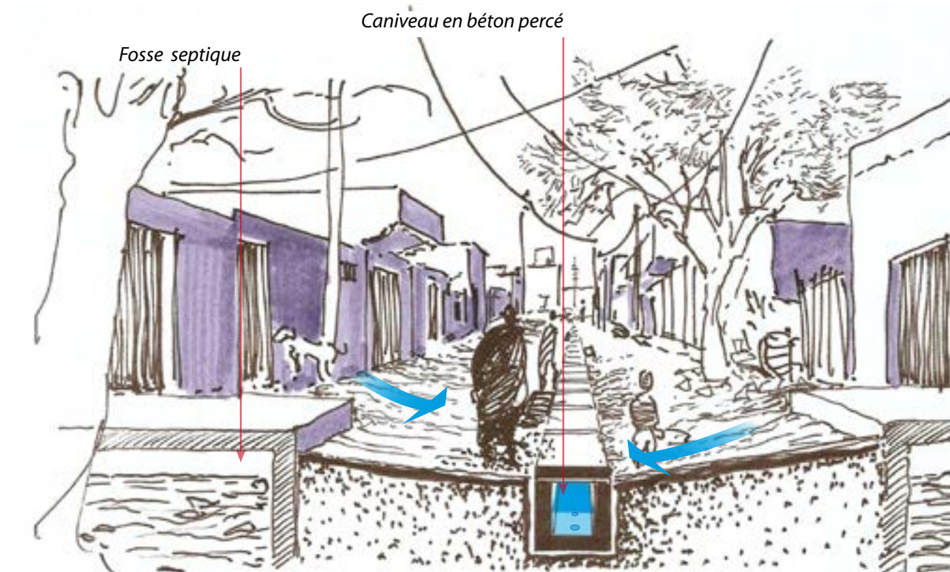
Dessin 1 Drainage des rues par des caniveaux en béton percé
